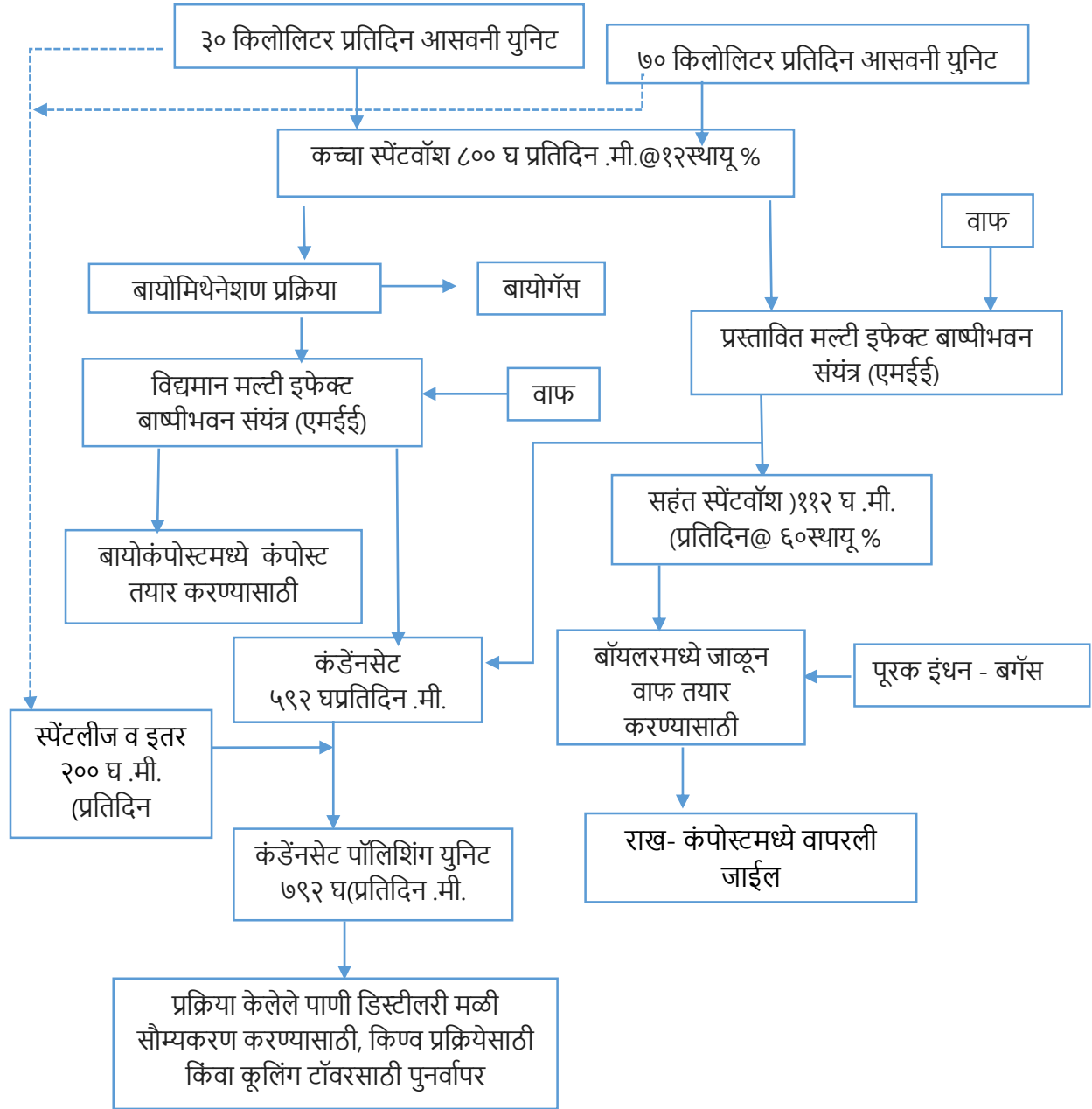
आकृती ९: आसवनी: स्पेंटवॉश प्रक्रिया व विल्हेवाट
