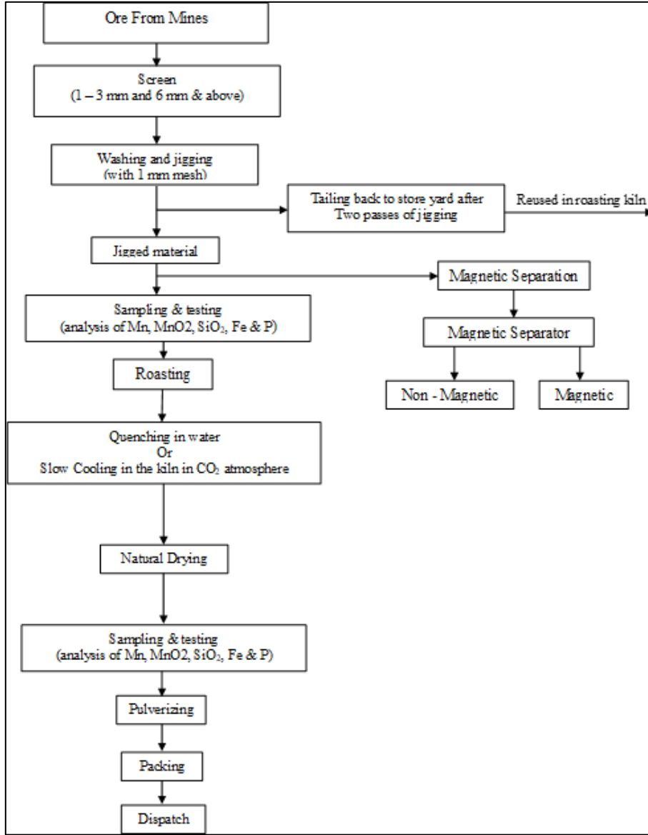
आकृती क्र. ४: मॅंगनीज डायऑक्साइड ते मॅंगनीज ऑक्साइड ची प्रक्रिया दर्शवणारा आराखडा
